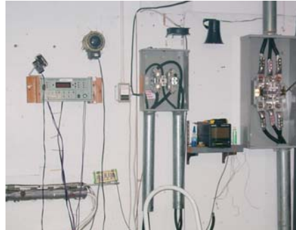
UL 414 Meter Socket Test Center
